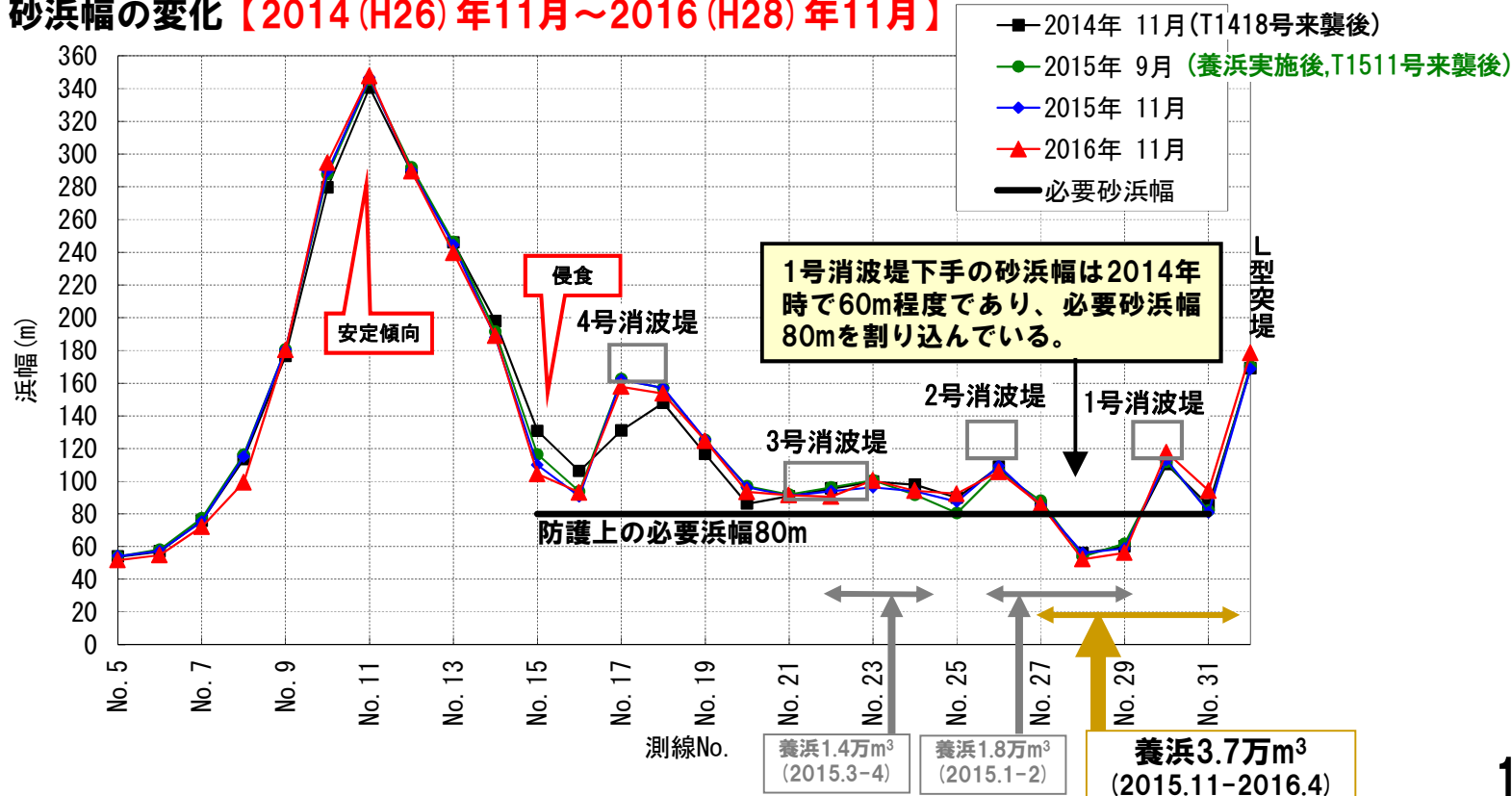
砂浜幅の変化【2014 (H26) 年11月～2016 (H28) 年11月】
